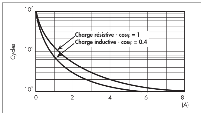
F 50 - Durée de vie électrique (AC) en fonction de la charge
