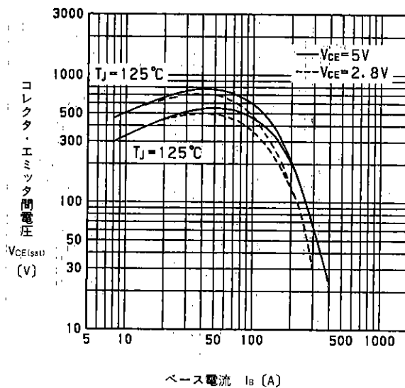
出力特性
