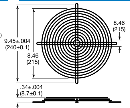
MG-200 (225 mm Fans)
