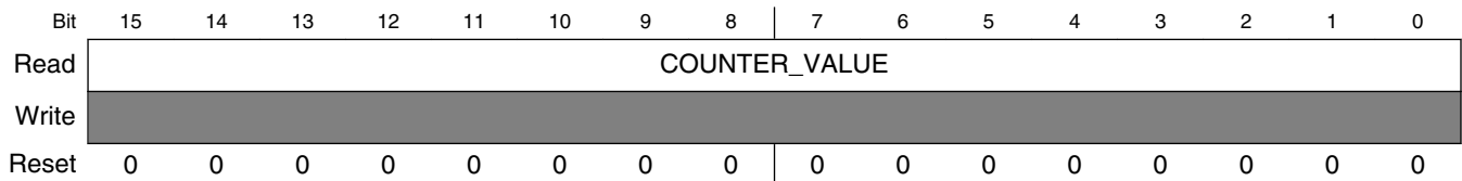
PITx_CNTR field descriptions
