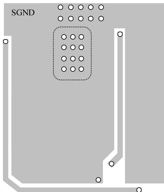
Bottom Layer
