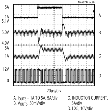
OUT5 LOAD TRANSIENT
