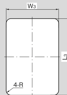
パネル穴明け寸法 Panel drilling dimensions
