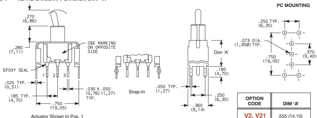
7101MD9_BE SPDT
