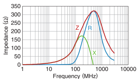
MMZ1608Q121B
