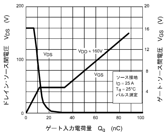
図 8.12 ダイナミック入出力特性
