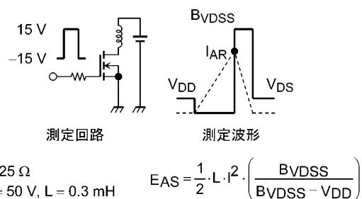
図 8.16 測定回路/測定波形
