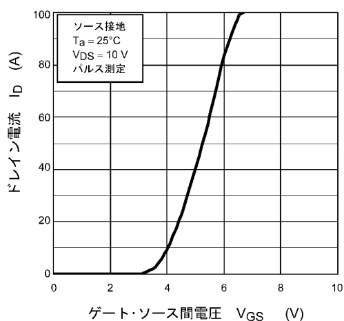
図 8.3 I_D - V_{GS}
