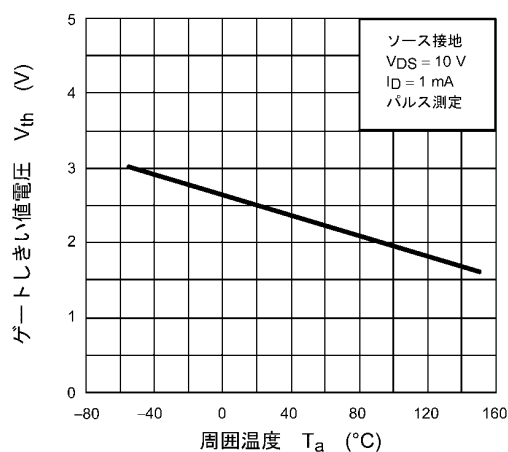
図 8.10 V_{th} - T_a
