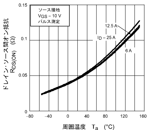
図 8.7 R_{DS(ON)} - T_a
