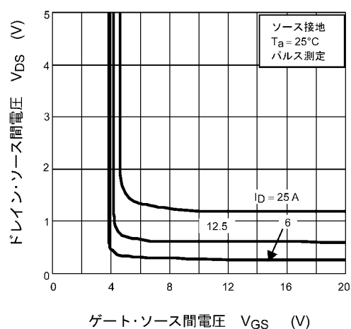
図 8.4 V_{DS} - V_{GS}
