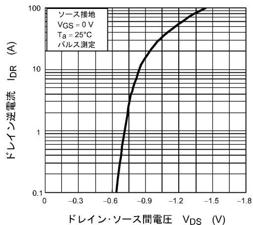
図 8.8 I_{DR} - V_{DS}
