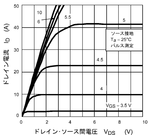
図 8.1 I_D - V_{DS}
