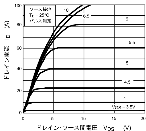
図 8.2 I_D - V_{DS}
