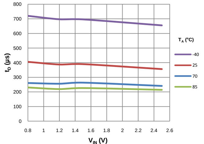
t_D vs V_{IN} , V_{BIAS}=2.5\text{V} ( C_{IN}=1\mu\text{F} , C_{SS}=1\text{nF} , R_L=10\Omega , C_L=0.1\mu\text{F} )
