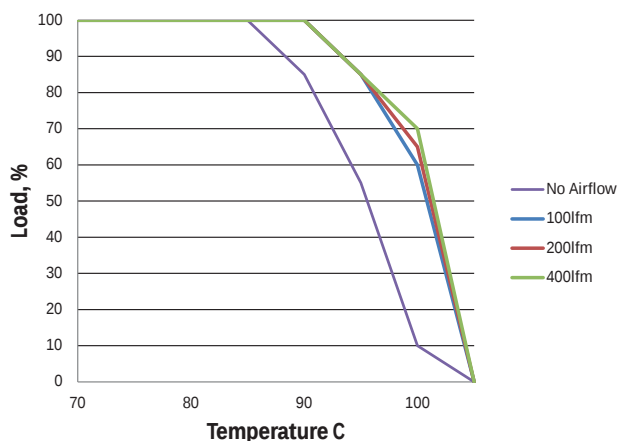
MTC2S1203MC - 18Vin
