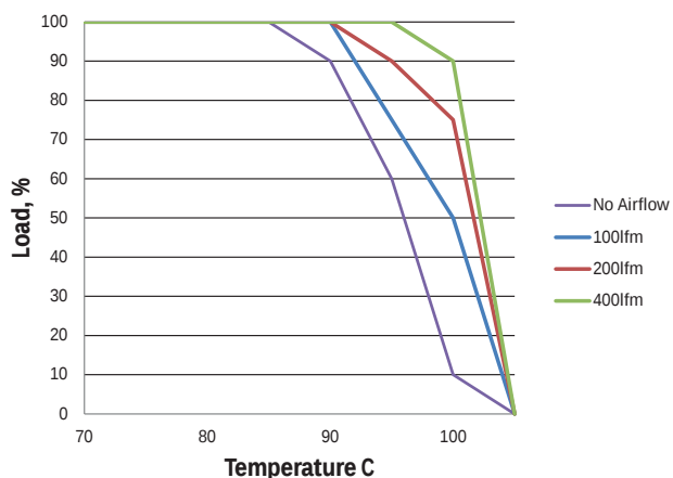
MTC2S1203MC - 9Vin
