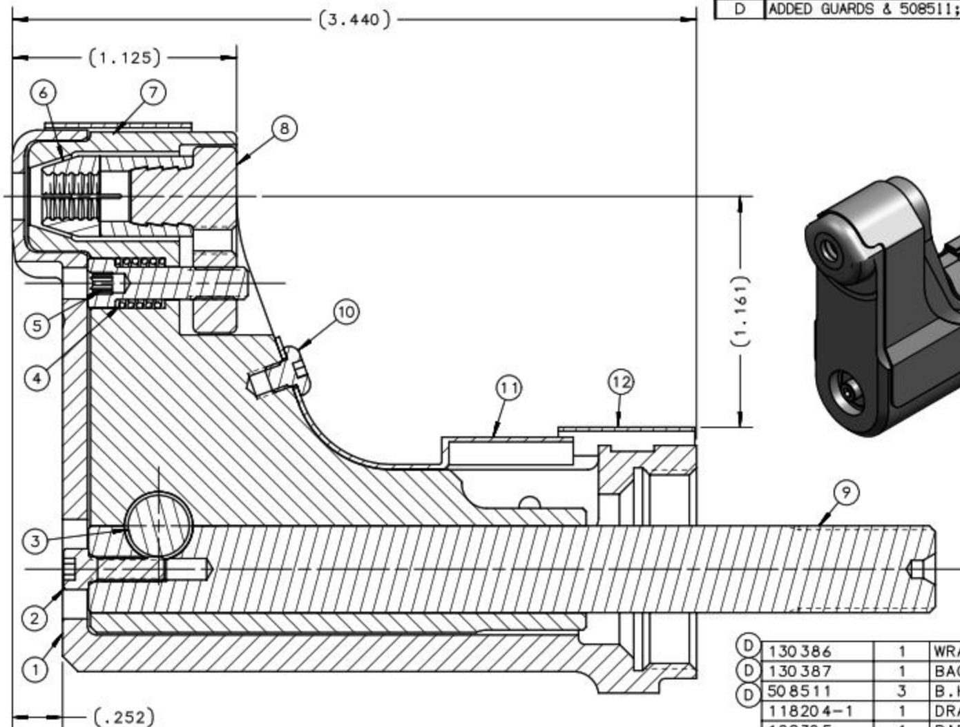
SECTION A-A
