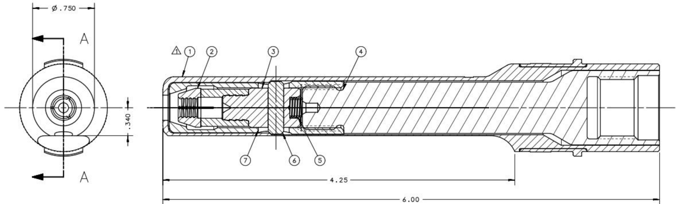
SECTION A-A
