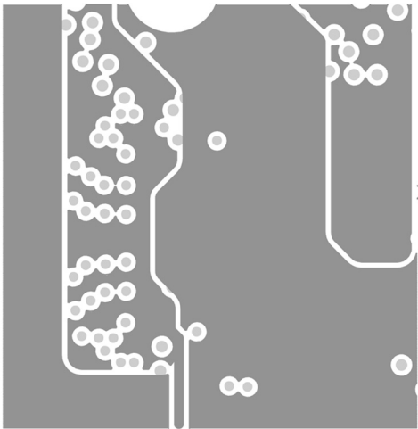
Inner Layer 5
