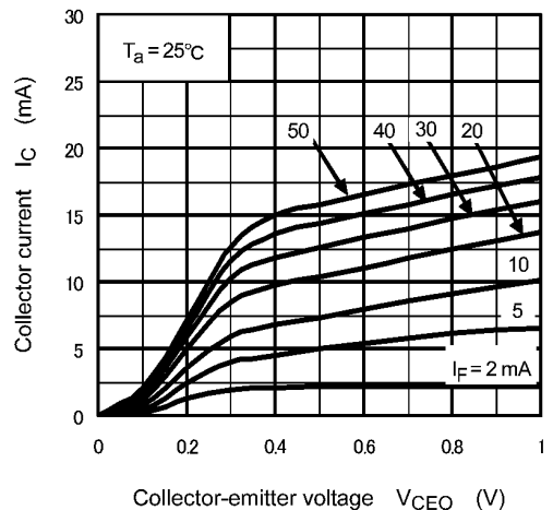
Fig. 11.8 I_C - V_{CE0}
