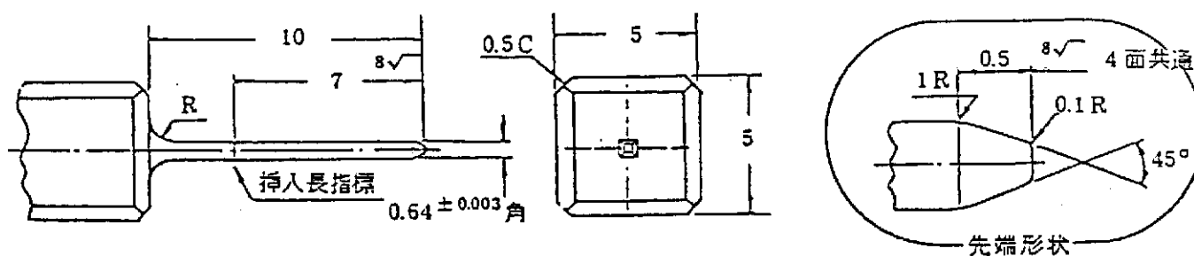
FIG-4 コンタクト挿抜力測定用ゲージ
