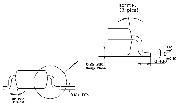
5-Pin TSOT (BD5)
