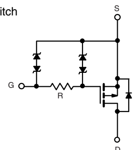
P-Channel MOSFET
