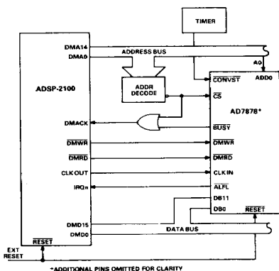
Figure 18. AD7878-ADSP-2100 Interface
