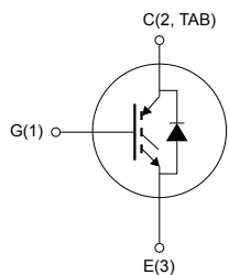
D 2 PAK
