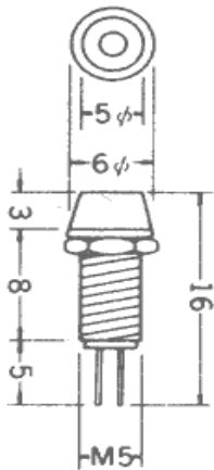
Model 407 ( 2 Volt ) 6 mm panel hole
