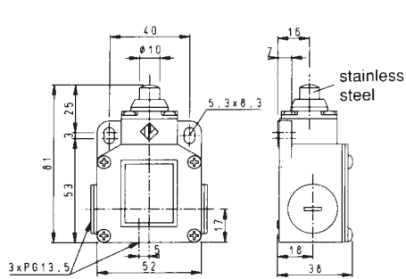
Actuator type 01 Piston plunger
