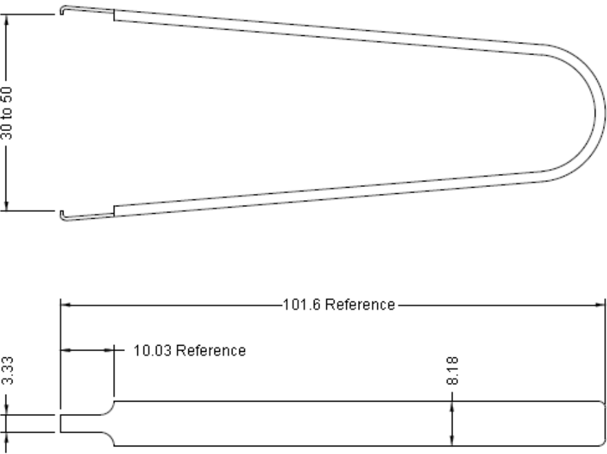
Dimensions : Millimetres
