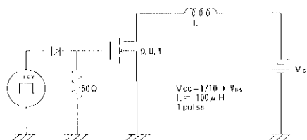
図1 測定回路
