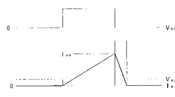
図2 動作波形
