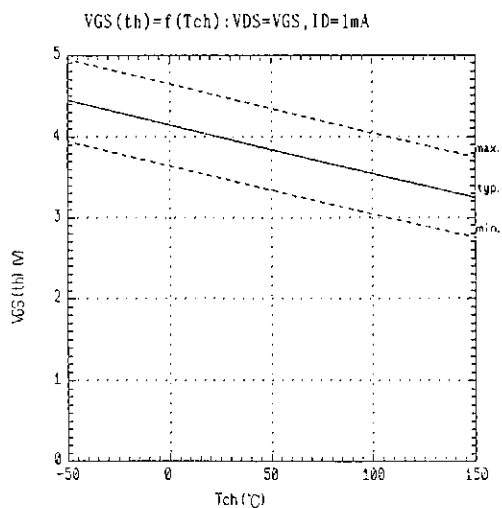
ゲートしきい値電圧 Gate threshold voltage
