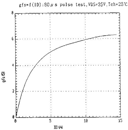
伝達コンダクタンス Typical transconductance
