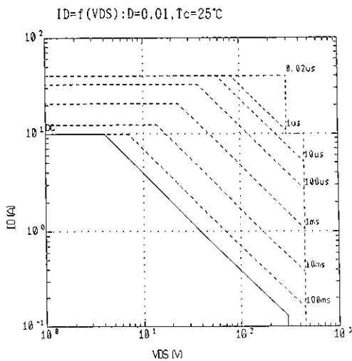
安全動作領域 Safe operating area
