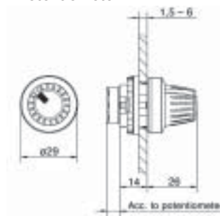
Potentiometer
