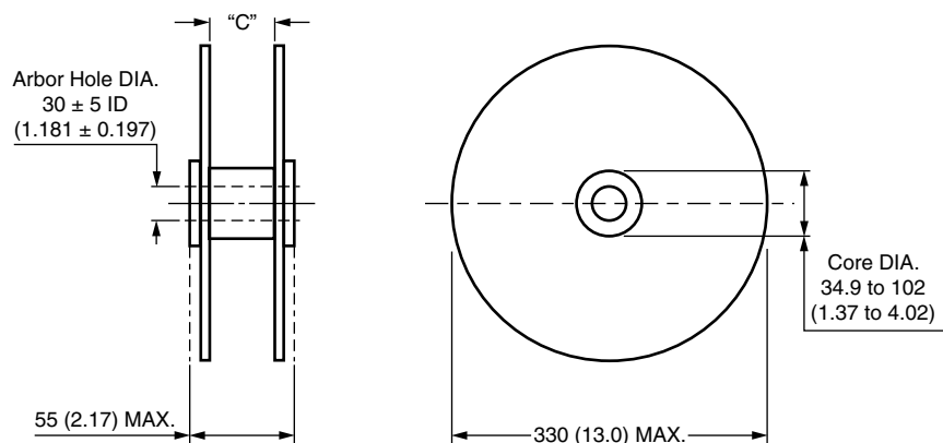
Fig. 7 - Reel Dimensions
