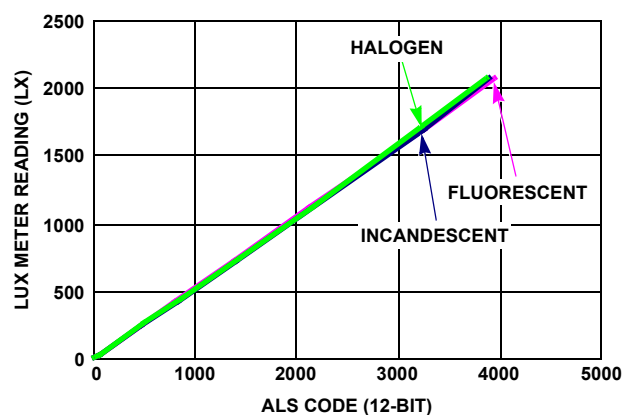
FIGURE 9. ALS LINEARITY OVER 3 LIGHT SOURCES (2000 LUX RANGE)
