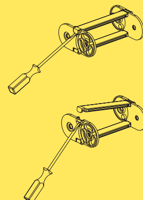
Rahmensteg montieren
