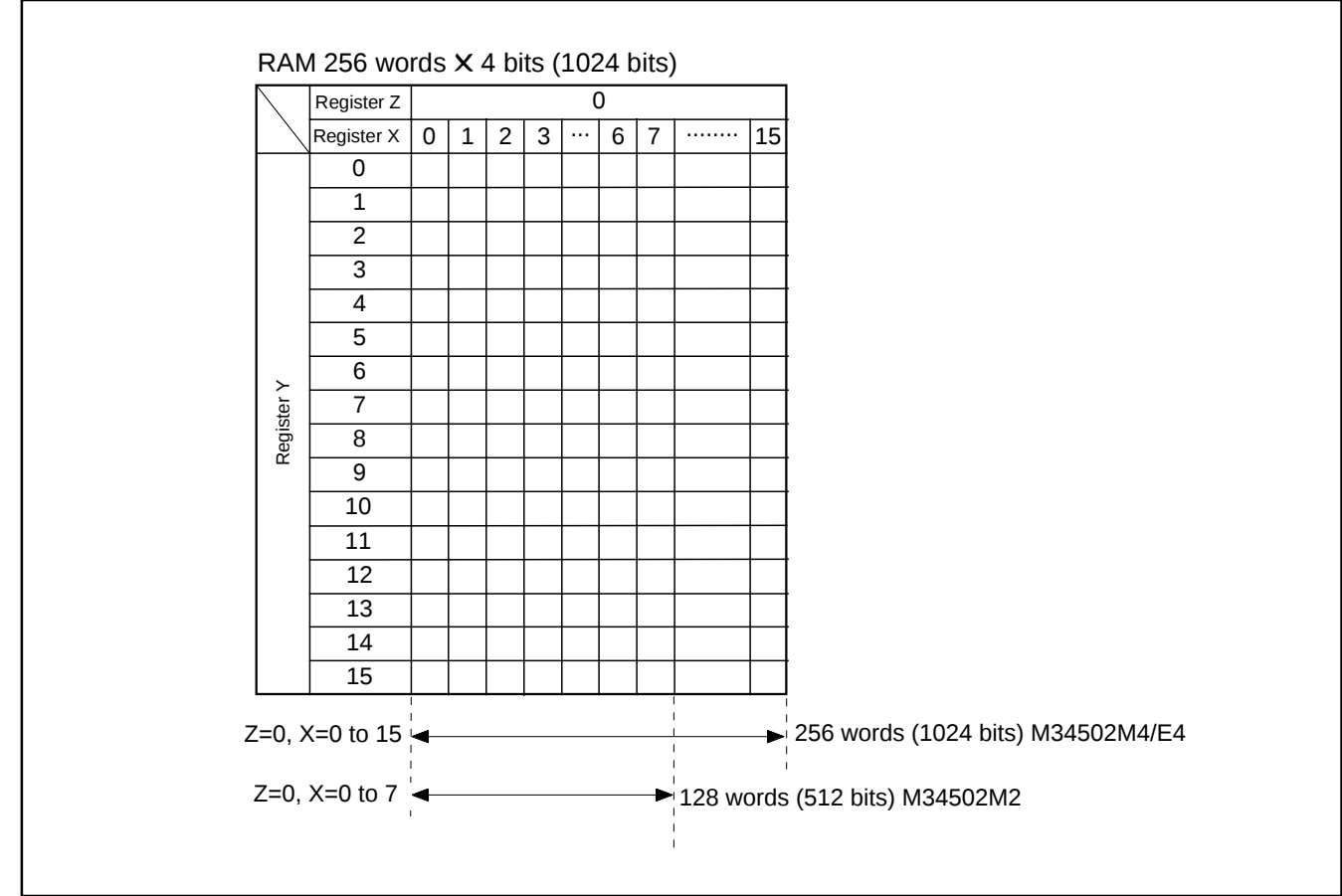
Fig. 12 RAM map
