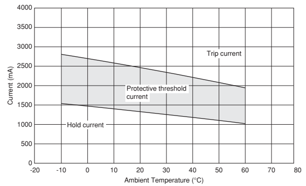
PTGL12AR0R2M1B51B0
