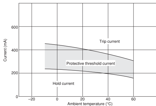
PTGL12AR150H8B72B0
