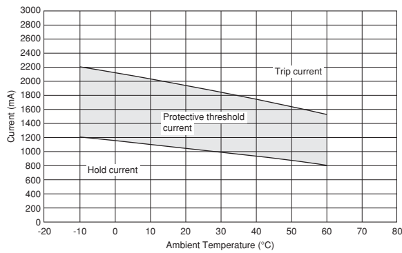
PTGL10ARR27M1B51B0
