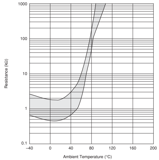
PRF15BG102RB6RC
