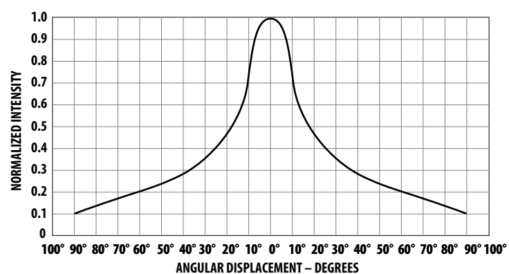
Figure 9: HLMP-Q102/-Q152
