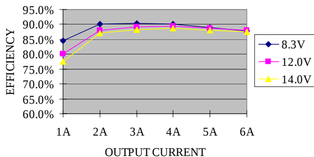
MODULE 2.5V
