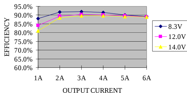
MODULE 3.3V
