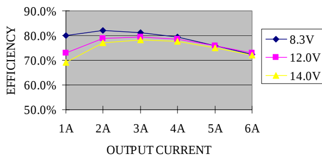
MODULE 0.75V
