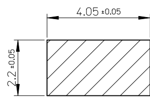
基板参考パターン P.W.B. PATTERN DIMENSION (REFERENCE)
