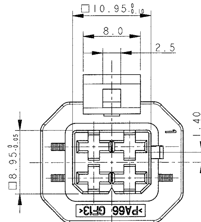
P/N 284677-1 NATURAL COLOR AS SHOWN (COLORE NATURALE COME MOSTRATO)
