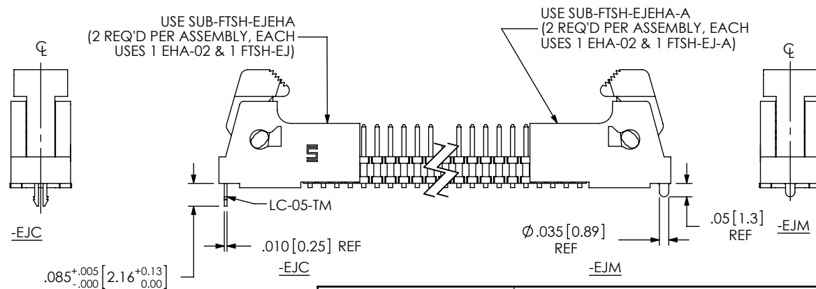
FIG 5 SCALE 2 : 1 -EJC & -EJM OPTIONS
