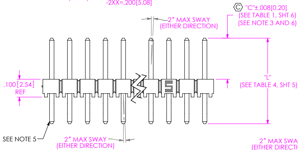
FIG 1 (TSW-1XX-XX-XX-S SHOWN)
