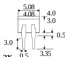
PS2505-2X PS2505-2
