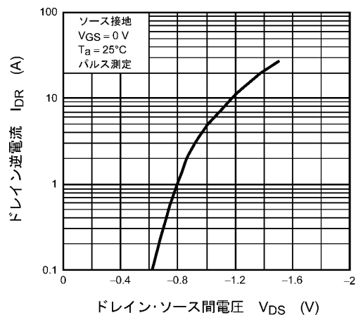
図 8.8 I_{DR} - V_{DS}
