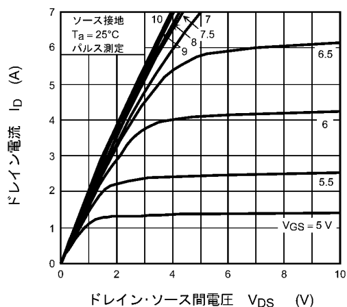
図 8.1 I_D - V_{DS}
