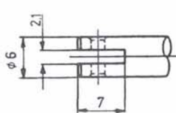
Ankerdetail
