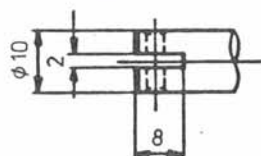
Ankerdetail
