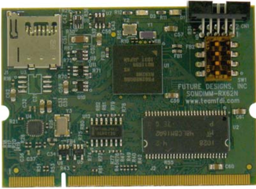
Actual PCB dimensions are 2.66" x 1.89"
