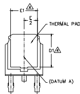
VIEW A-A
