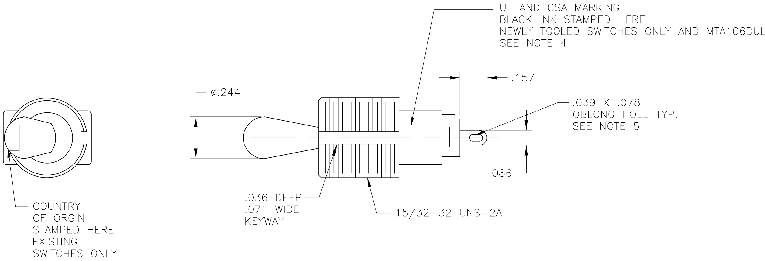
WIRE LUG TERMINAL
