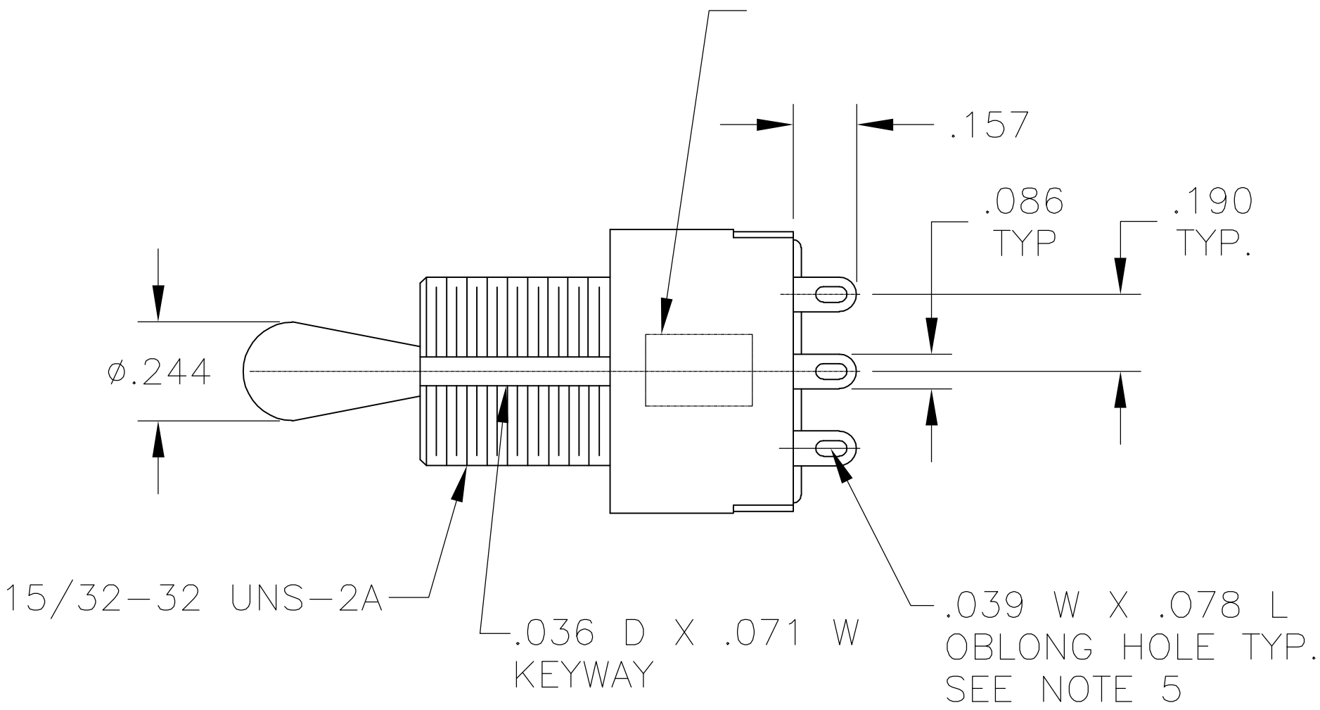
WIRE LUG TERMINAL
