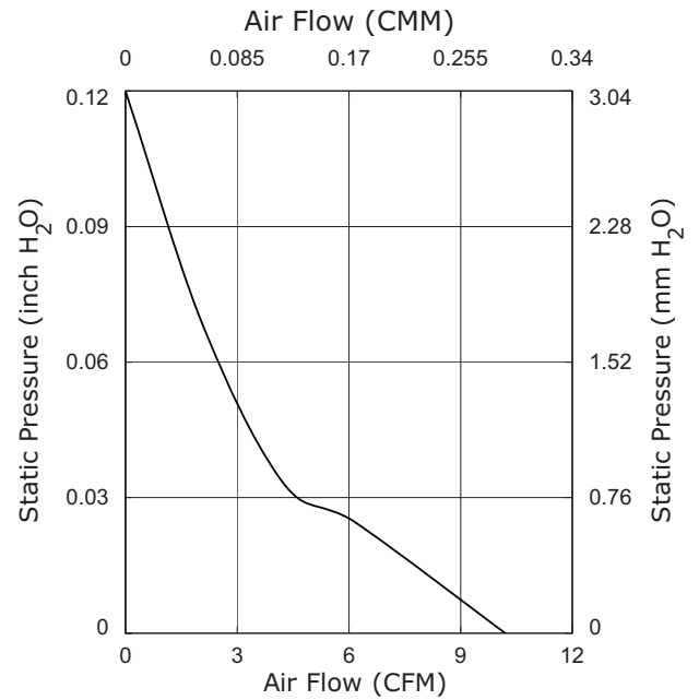
CFM-5015V-138-201
