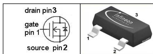
PG-SOT-23
