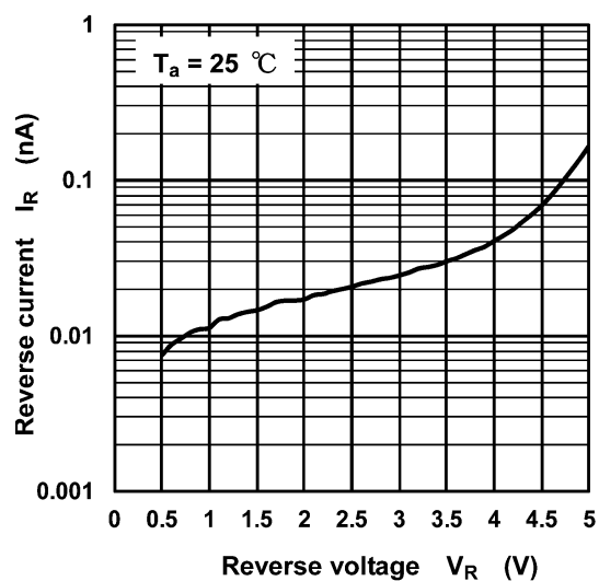
図 8.2 I_R - V_R
