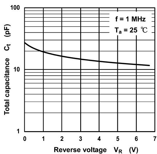
図 8.3 C_t - V_R
