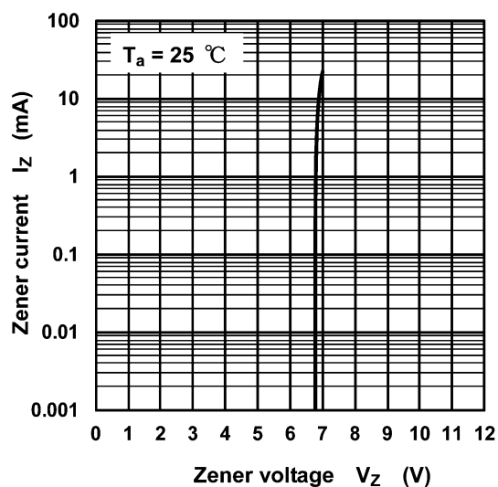
図 8.1 I_Z - V_Z
