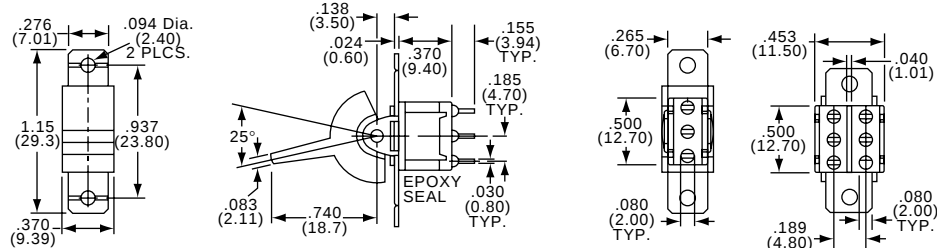
SPDT
