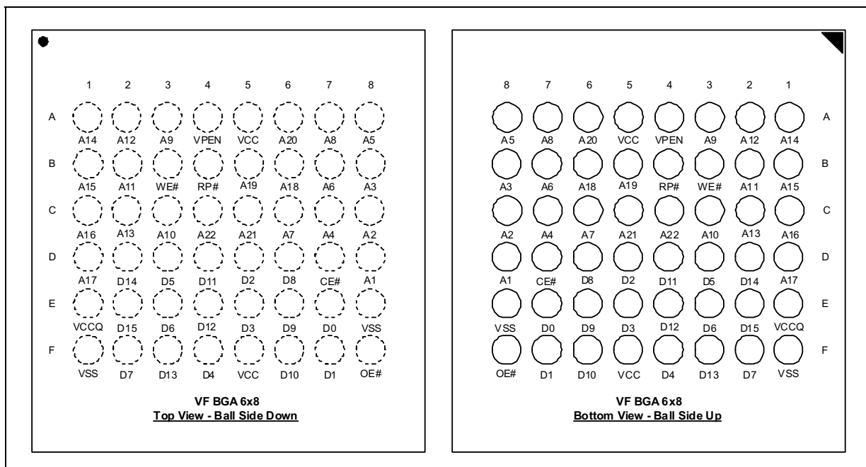
Figure 3. 3 Volt Intel StrataFlash® Memory VF BGA Ballout(32 Mbit)
