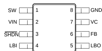
DU PACKAGE (Top View)
