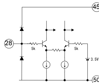
28: EHT in
