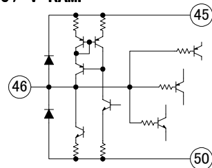
46: V RAMP
